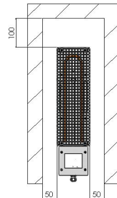
Anschlusskasten unten (Eine Montage mit Anschlusskasten oben ist nicht zugelassen!)
