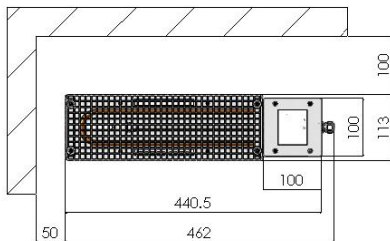
Anschlusskasten rechts Boîte de raccordement à droite
