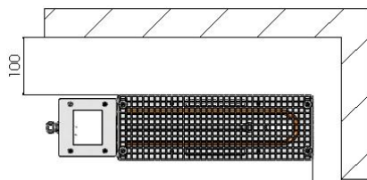
Anschlusskasten links Boîte de raccordement à gauche
