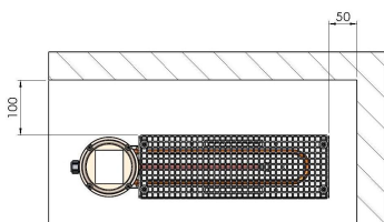
Anschlusskasten links Boîte de raccordement à gauche
